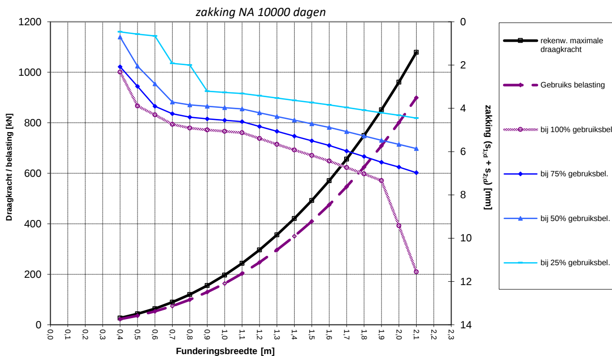
Figuur 5 Draagkracht-last-zakkingsgrafiek
