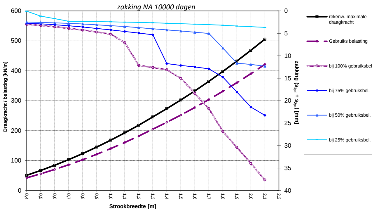
Figuur 3 Draagkracht-last-zakkingsgrafiek
