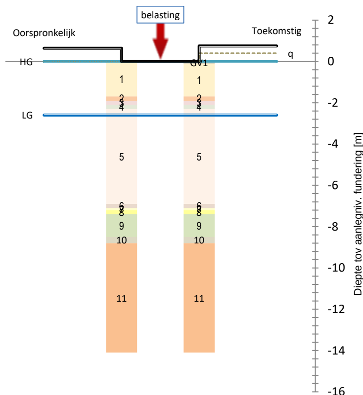
figuur 1.1 - Schematisatie van de bodemopbouw
